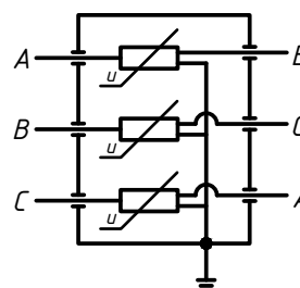
СХЕМА ПОДКЛЮЧЕНИЯ
